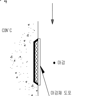
<그림 6.3.6> 재료분리 단면복구공법 개요도 및 시공순서
